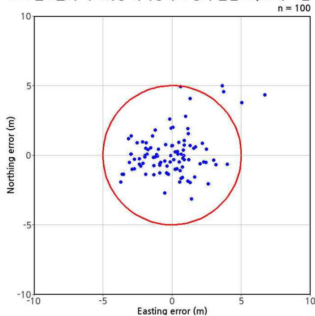
2025년 3분기 국토위성 위치정확도 평가 산점도 (24개 도엽 기준)
