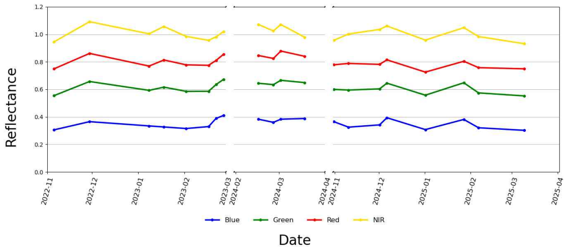
TDI 2(동절기)
