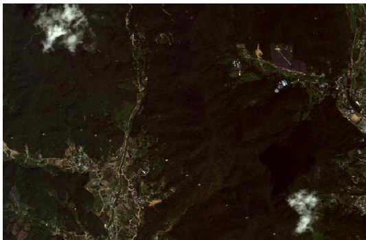
국토위성 칼라합성영상
