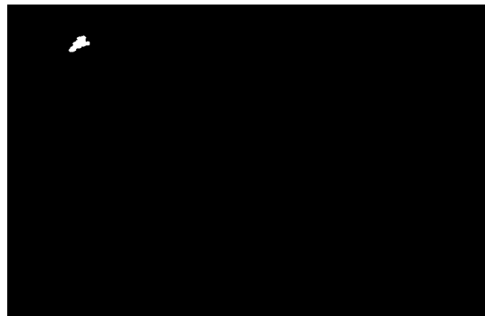
구름화소(흰색)
