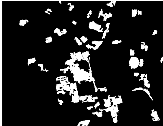
구름화소(흰색)
