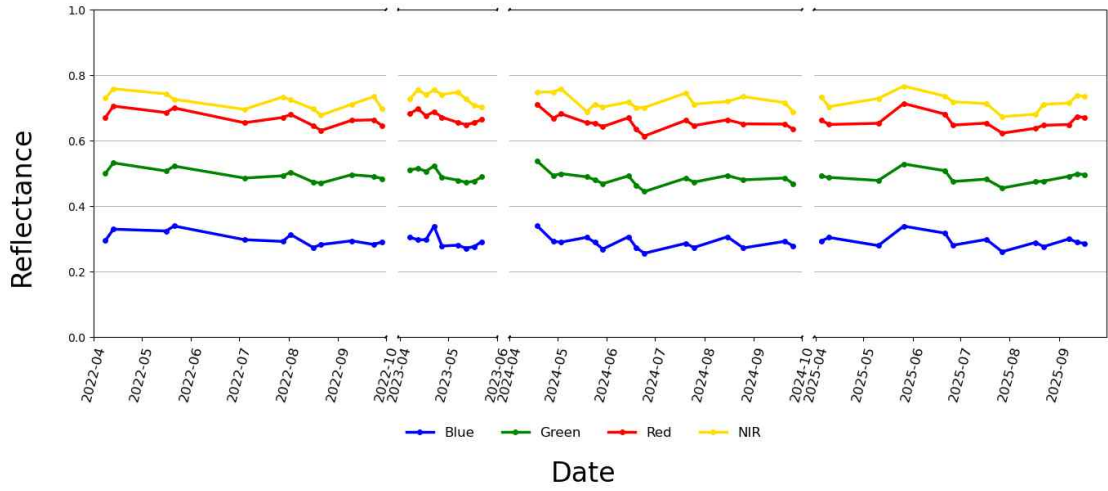
TDI 1(하절기)
