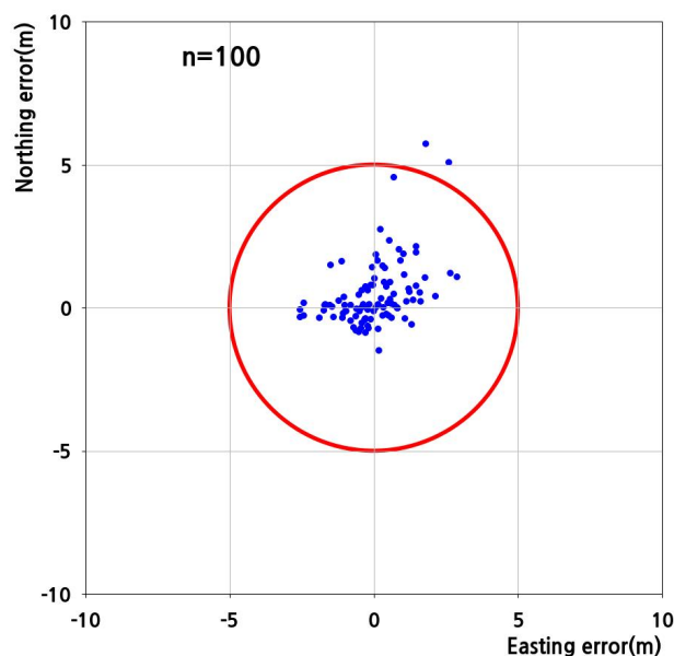
2024년4분기 국토위성 위치정확도 평가 scatter plot(24개 도엽기준)
