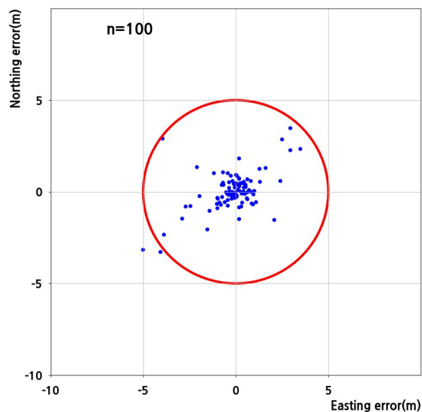
24년1분기 국토위성 위치정확도 평가 scatter plot(24개 도엽기준)
