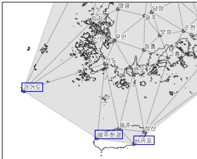
&lt;신규 위성기준점 설치시 Network-RTK 망 구성도&gt;
