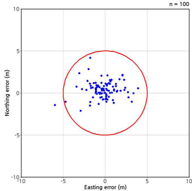
2025년 2분기 국토위성 위치정확도 평가 산점도 (24개 도엽 기준)
